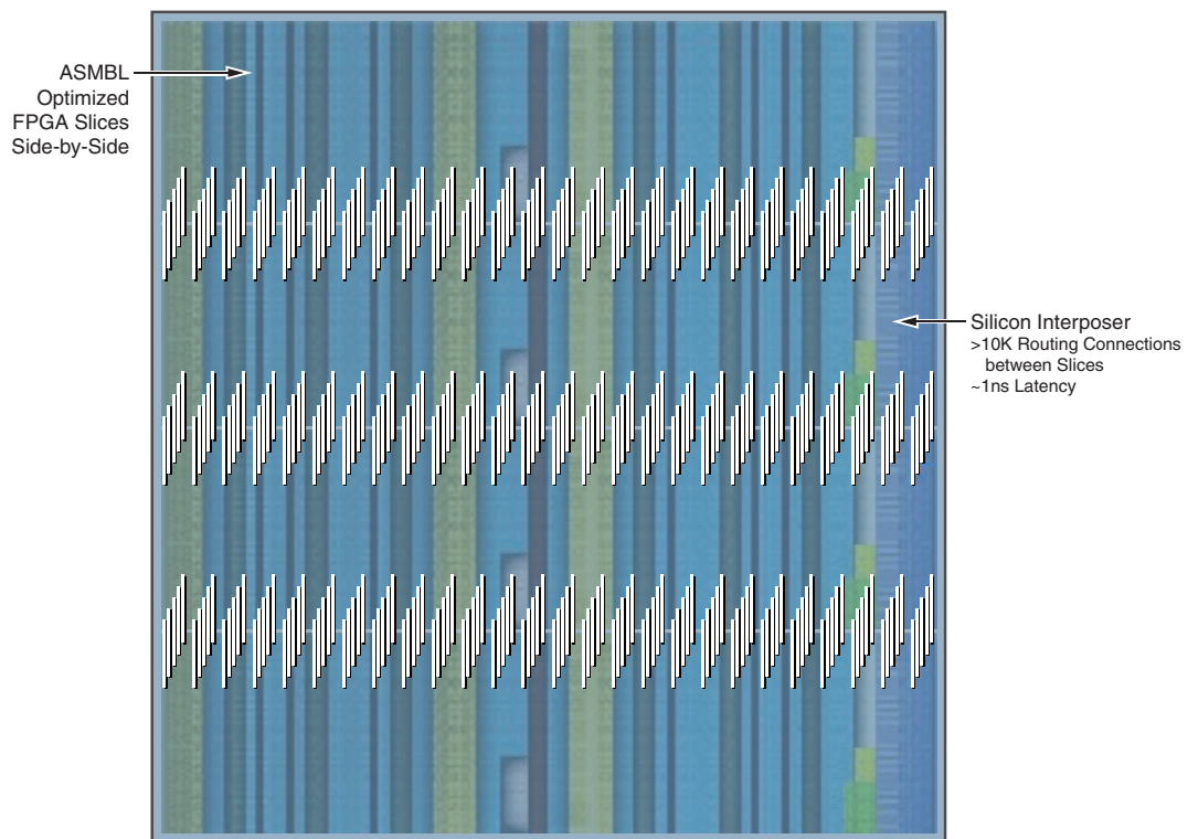
図 5 : アセンブリされたダイスタックの「X 線図」
