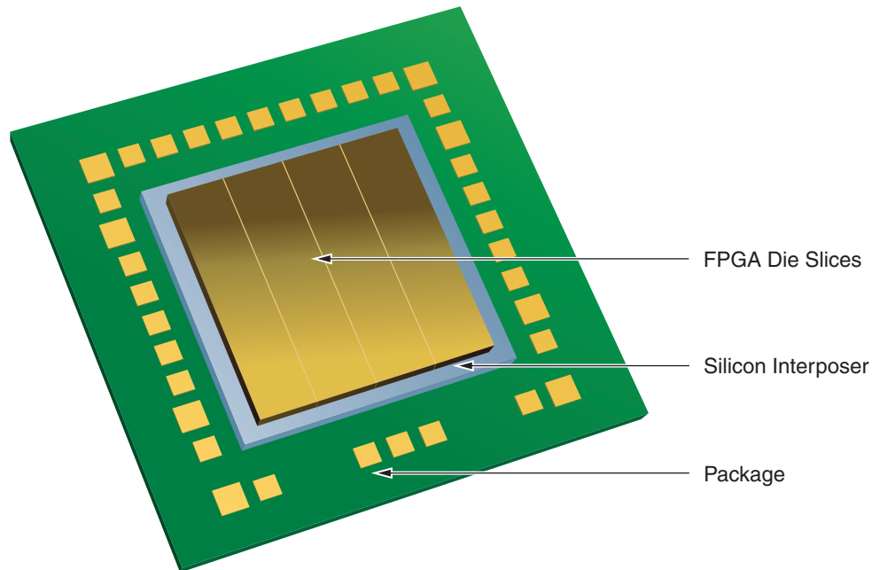
図 1: スタックド シリコン インターコネクト テクノロジーを適用して作成したダイの上面図
